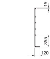
Typ GI
