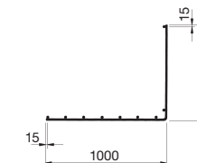
Typ AAL
